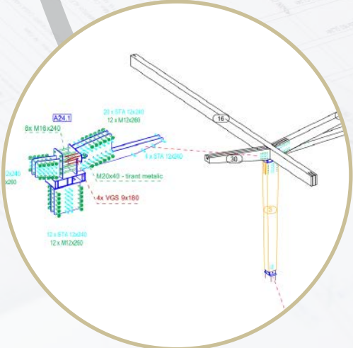
PLANURI MONTAJ
